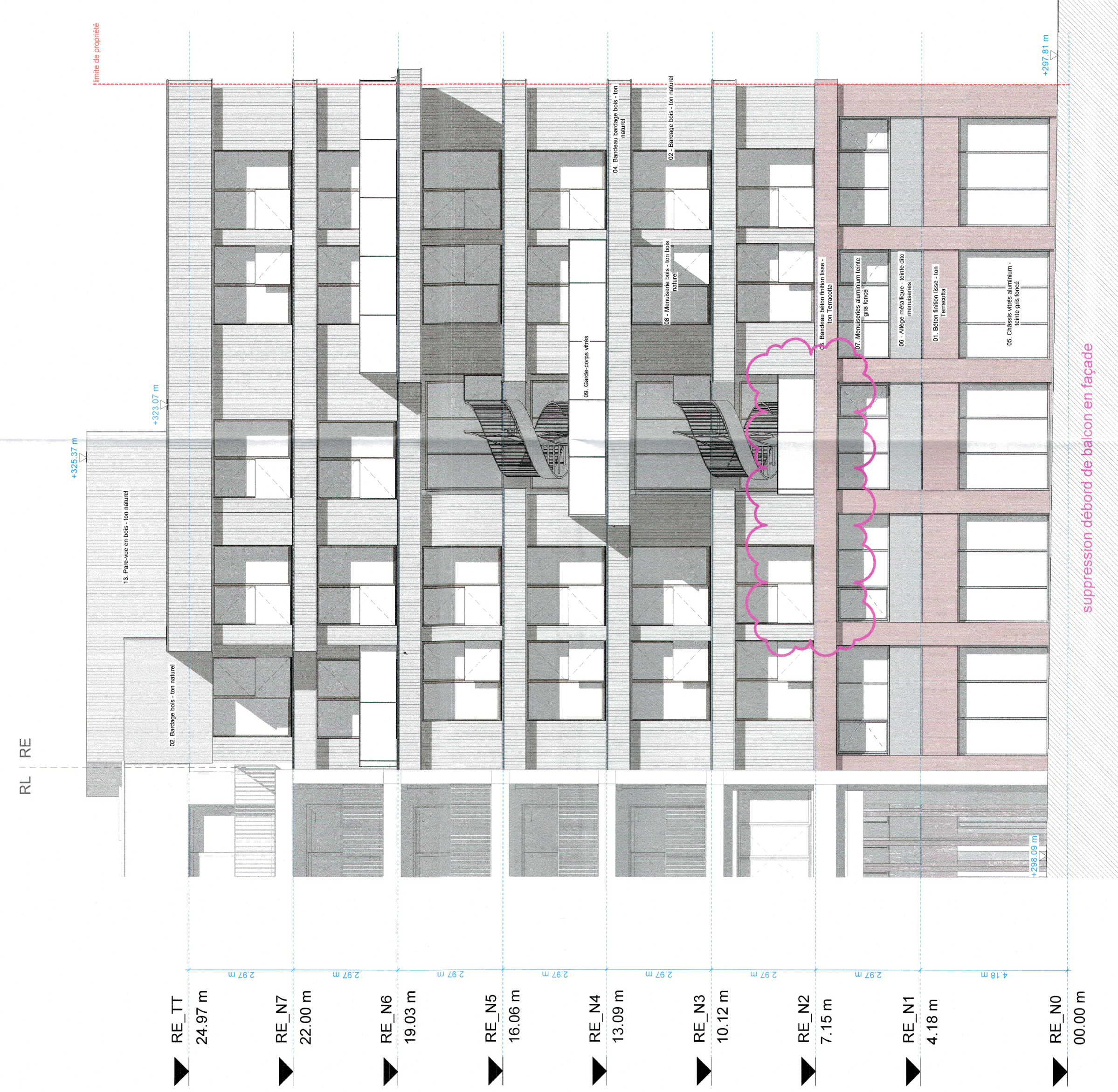
Elévation Oust 1:100
